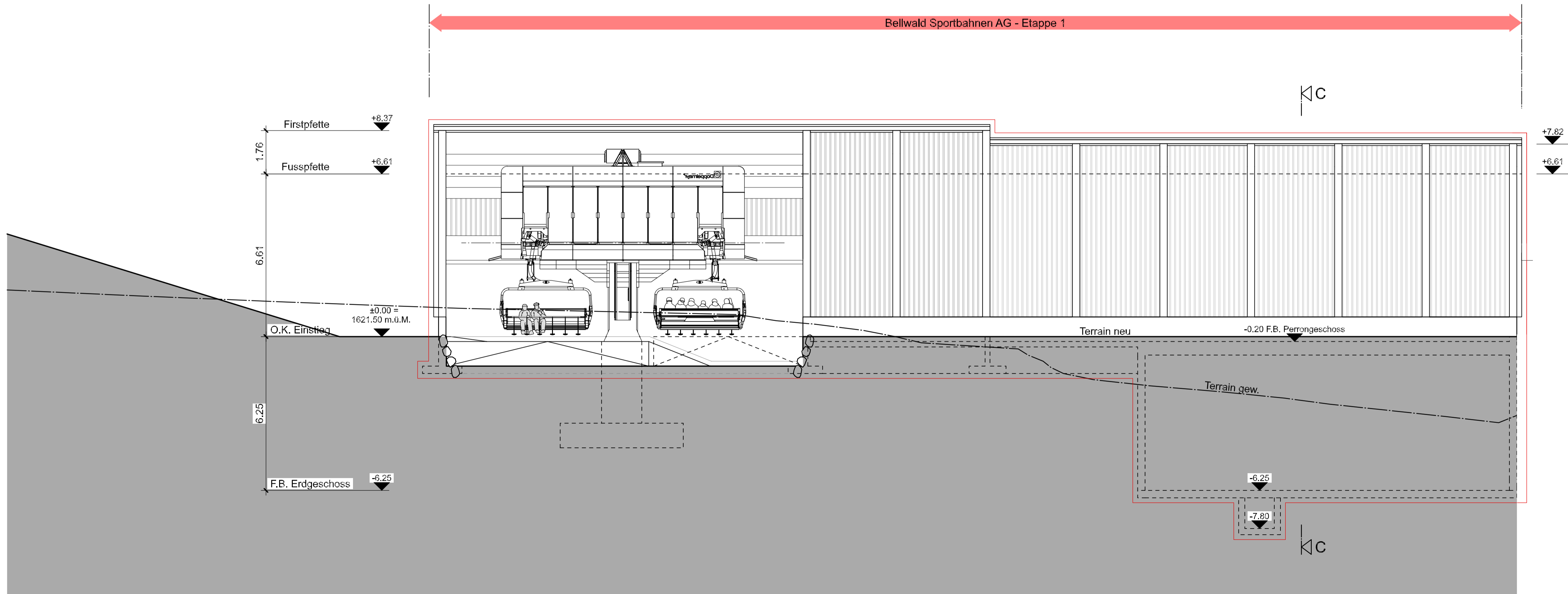
Fassade Nord Mst.: 1:100
