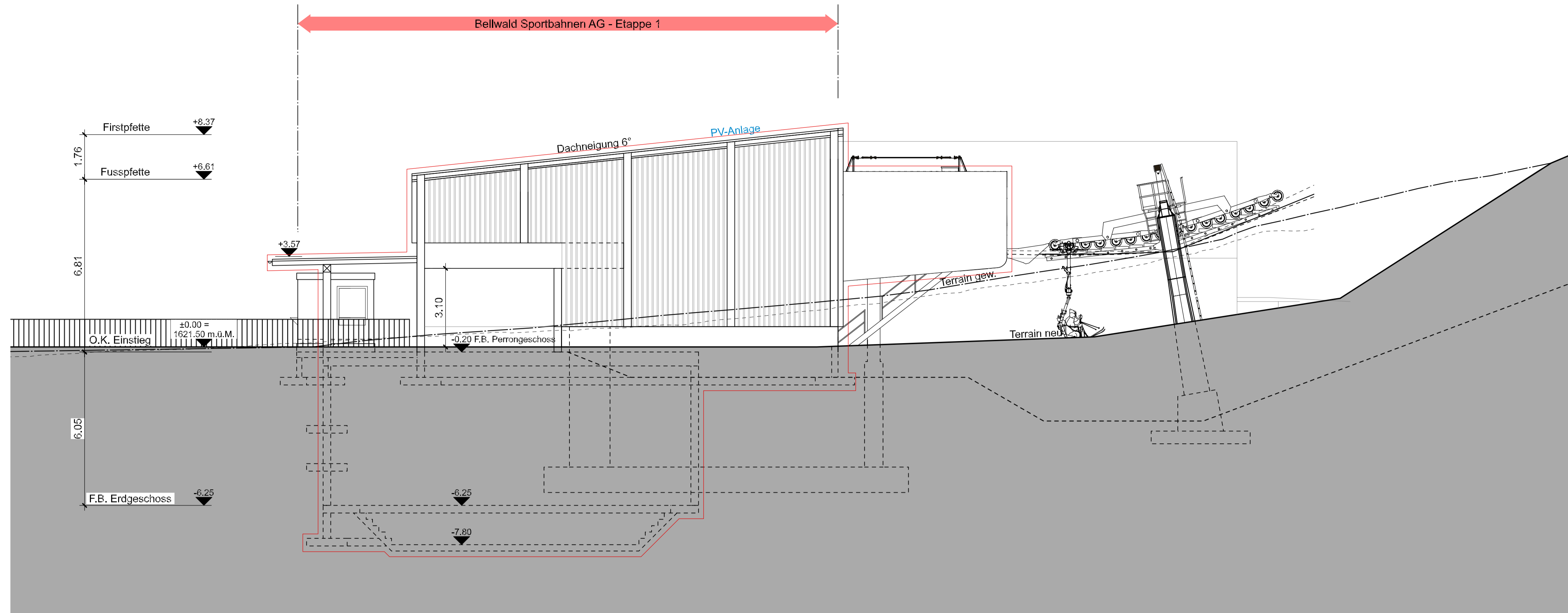
Fassade Ost Mst.: 1:100
