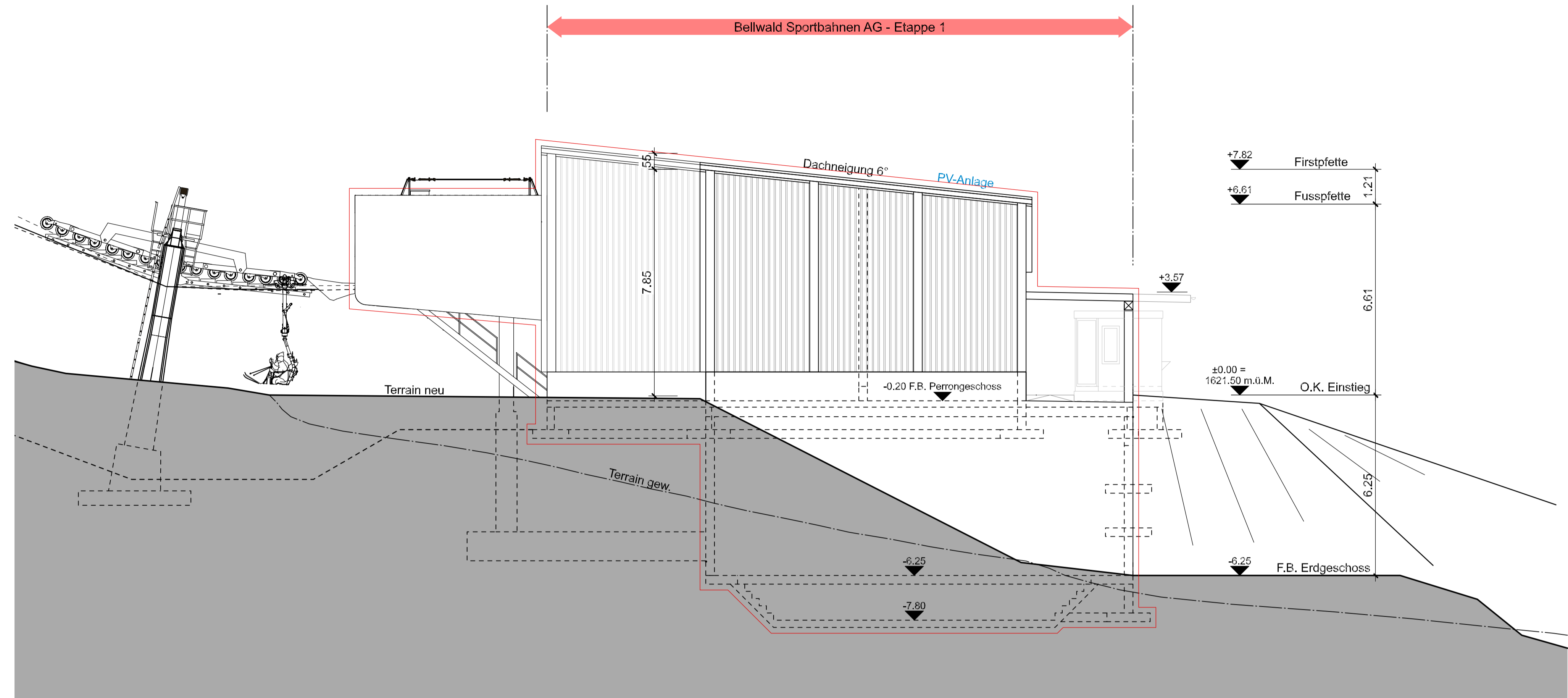
Fassade West Mst.: 1:100
