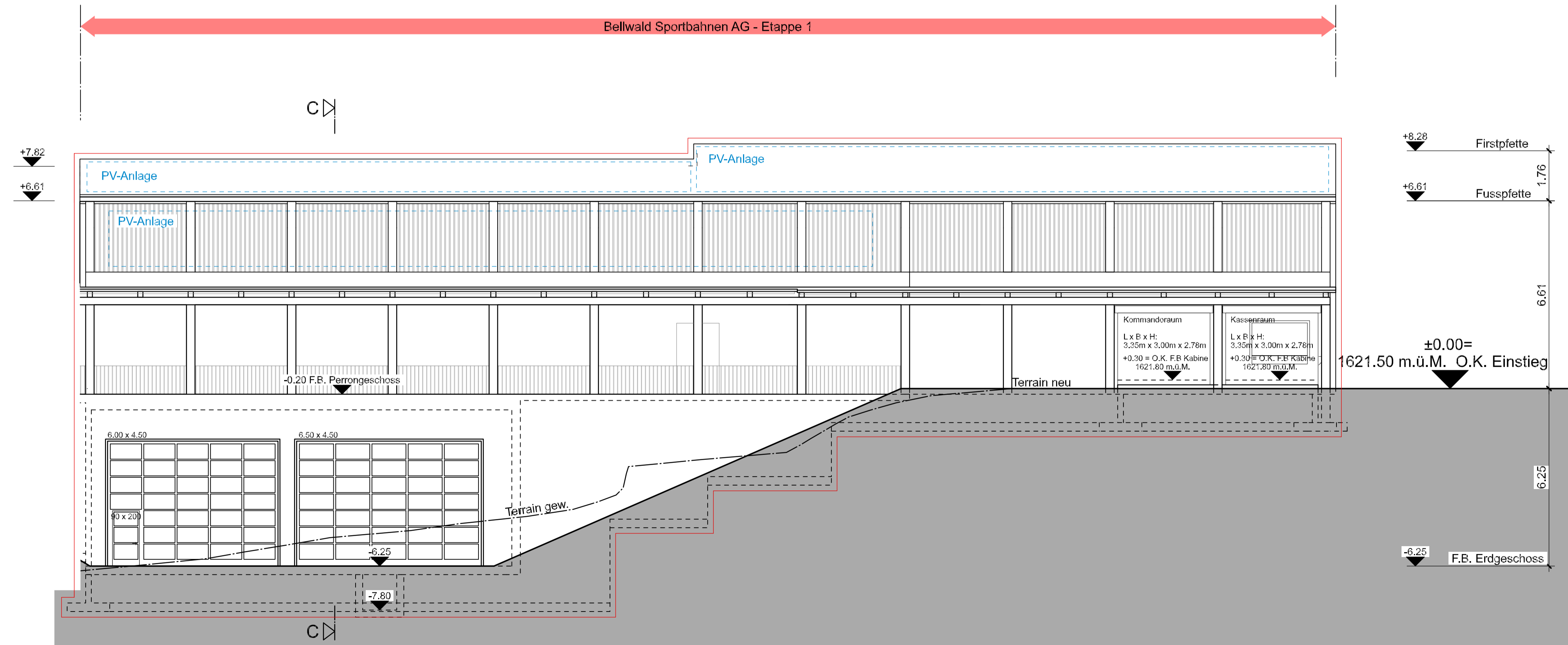
Fassade Süd Mst.: 1:100
