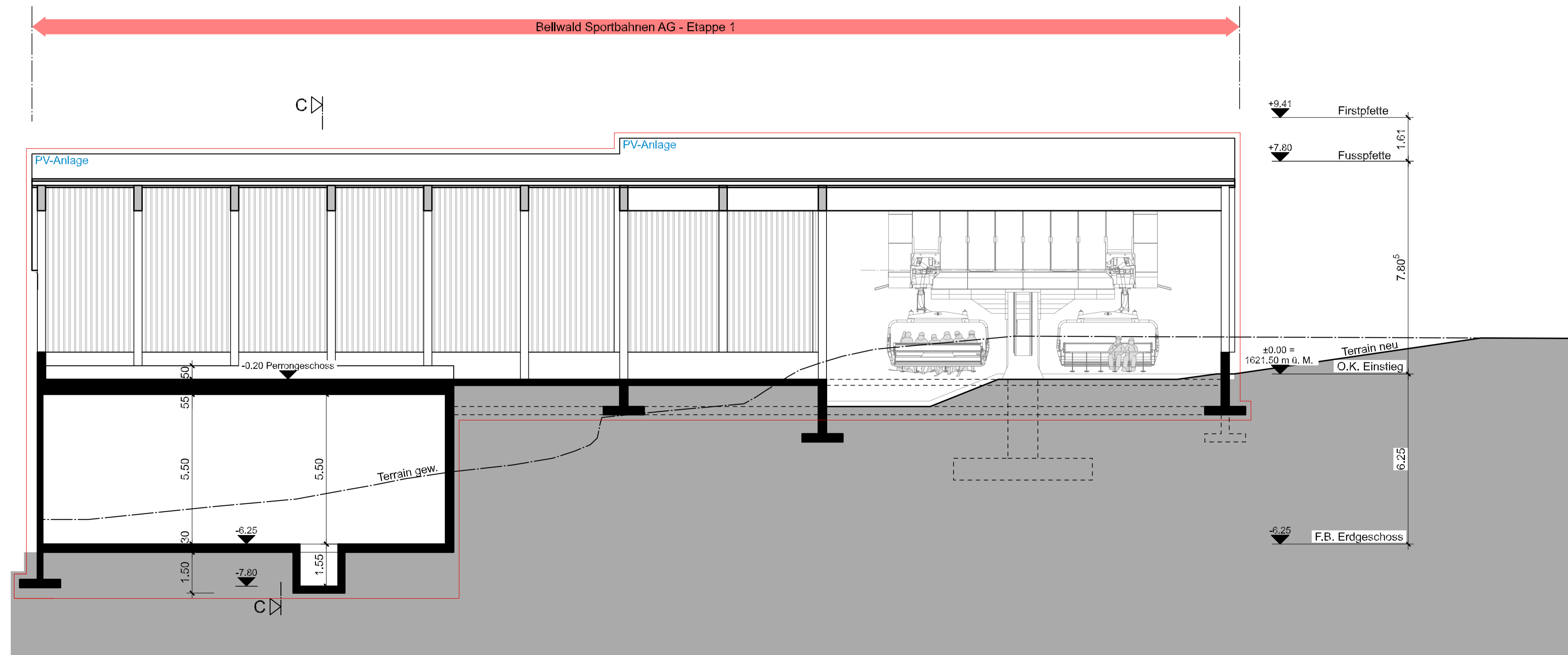
Schnitt A-A Mst.: 1:100
