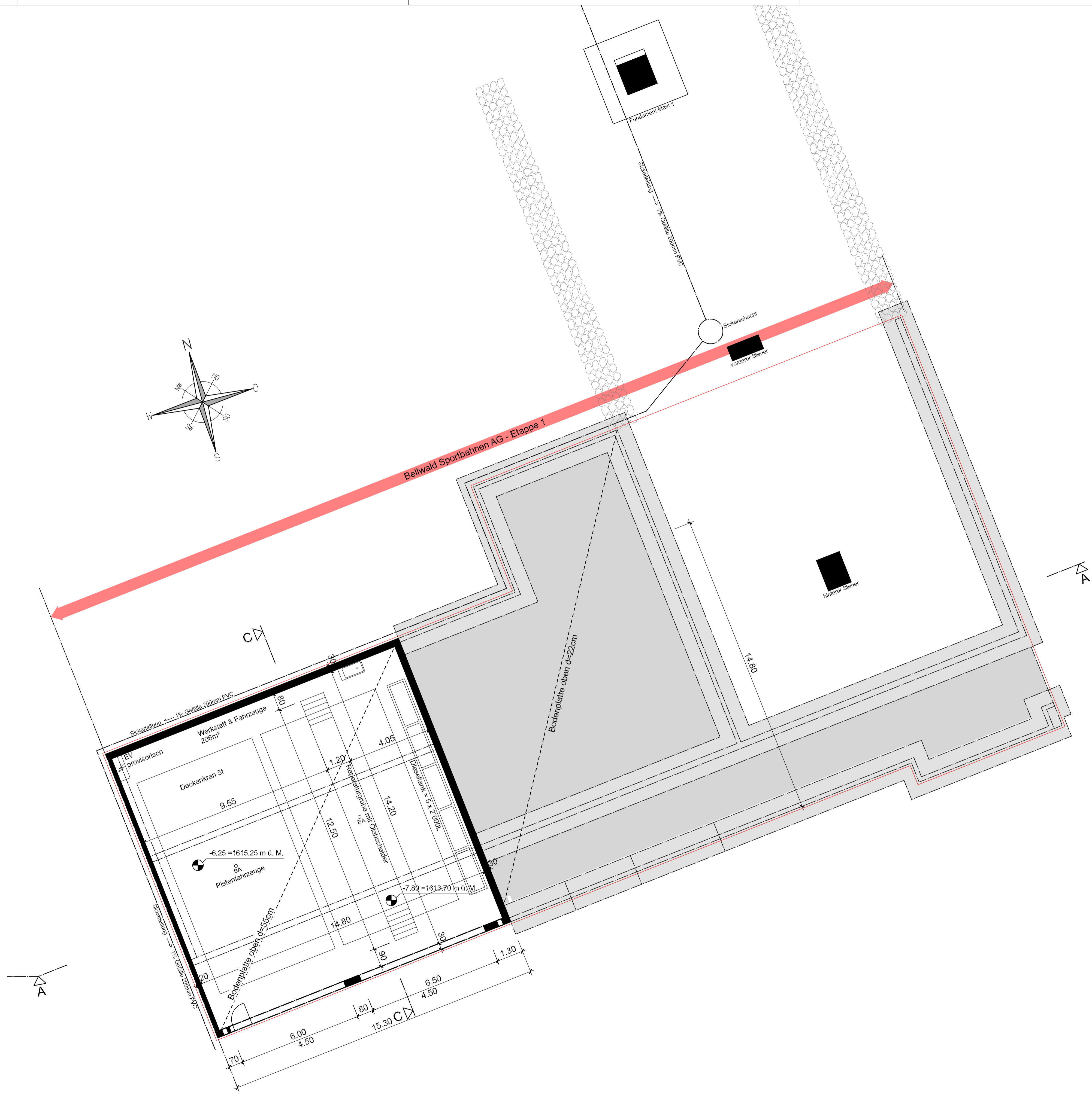
Grundriss Erdgeschoss Mst.: 1:100
